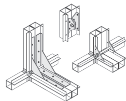
Schéma pripojenia sekcií
