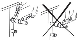
Pripojenie rúrok
