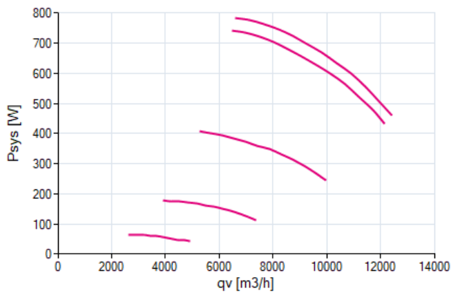
příkon P_{sys}
