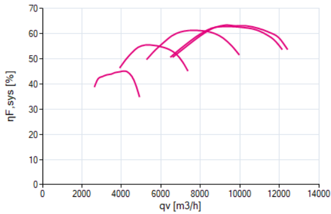
účinnost \eta_{F,sys}
