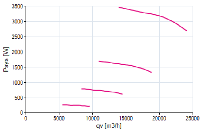
příkon P_{sys}
