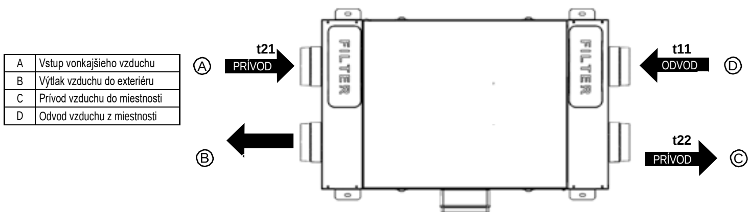
obr.7.a Teplotné čidlá
