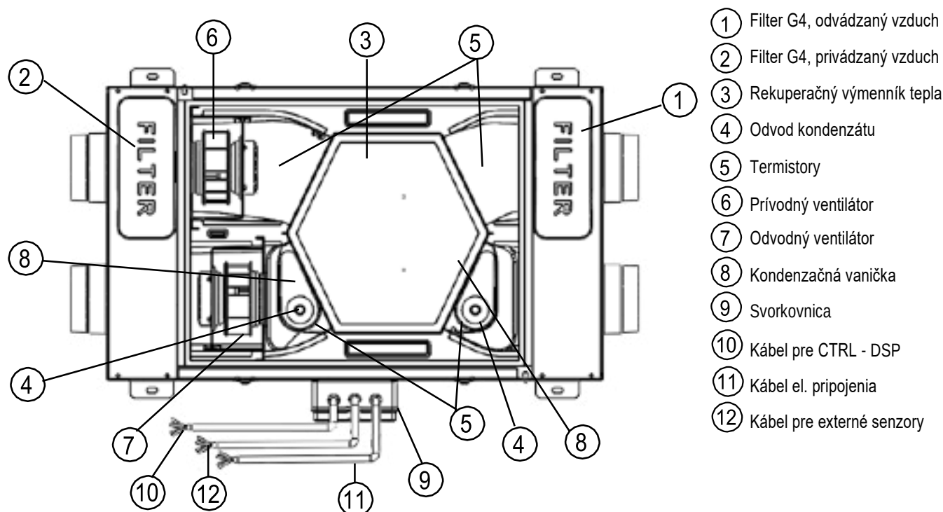
Obr. 8.a Vnútorne komponenty
