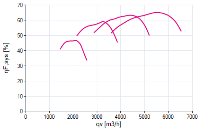
účinnost \eta_{F,sys}
