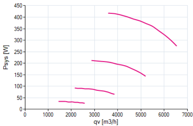
příkon P_{sys}
